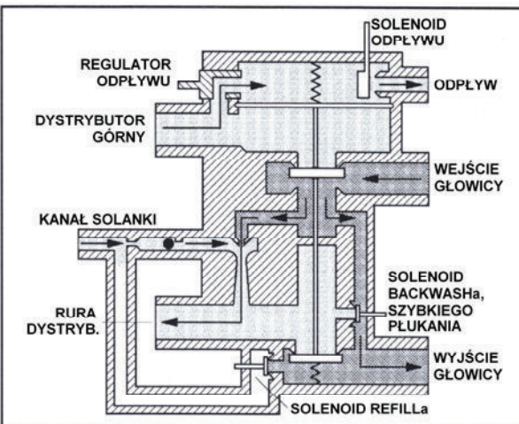
ZASSANIE SOLANKI/ WOLNE PŁUKANIE ZŁOŻA
