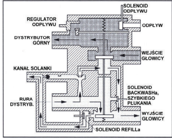
NAPEŁNIANIE ZB. SOLANKI
