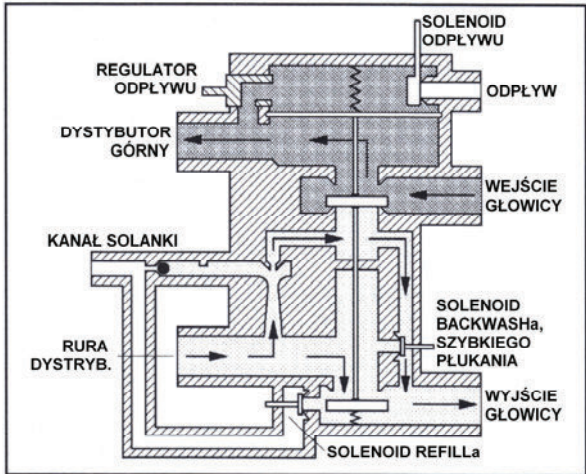
PRZYGOTOWANIE SOLANKI
