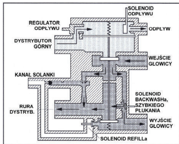
SZYBKIE PŁUKANIE ZŁOŻA (541N84)
