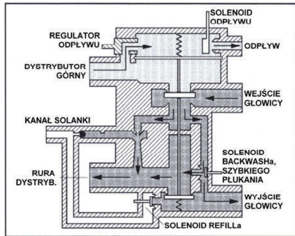
PŁUKANIE WSTECZNE (541N84)
