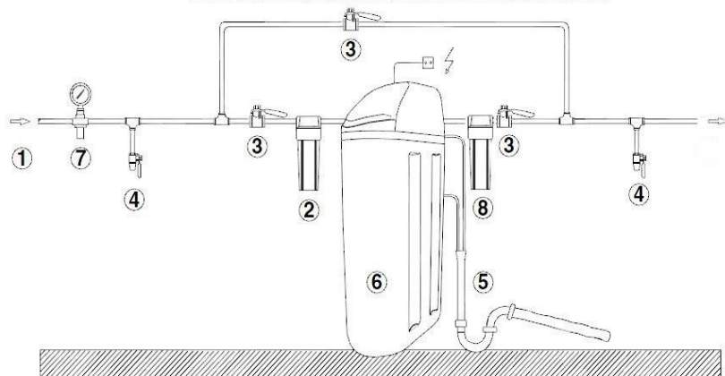
SCHEMAT PODŁĄCZENIA ZMIĘKCCZACZA / UZDATNIACZA WODY
