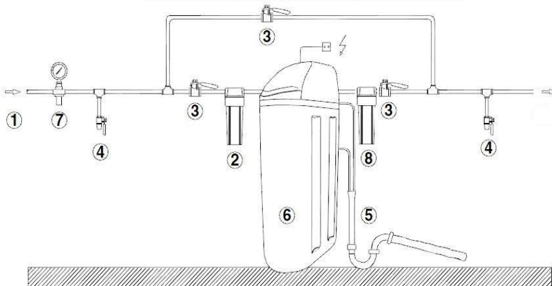
SCHEMAT PODŁĄCZENIA ZMIĘKZACZA / UZDATNIACZA WODY
